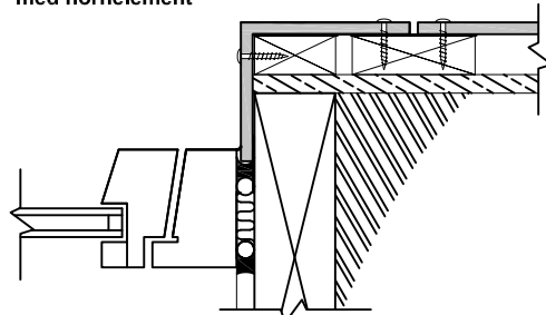
Horisontellt snitt exempel på fönster-lösning med hörnelement
