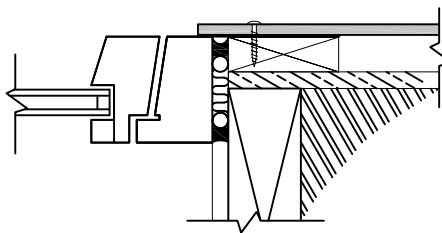
Horisontellt snitt exempel på fönster- lösning med plåt
