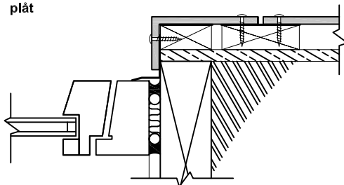
Horisontellt snitt exempel på fönster-lösning med fönster monterad i samme "liv" som fasad
