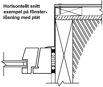
Horisontellt snitt exempel på fönster- lösning med plåt
